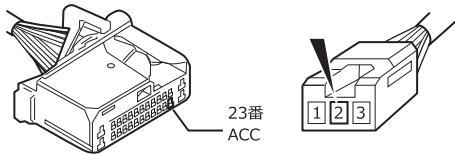
車両側ACC電源の配置 (24P)
